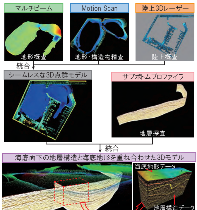
図1 一元化データ作成フロー
