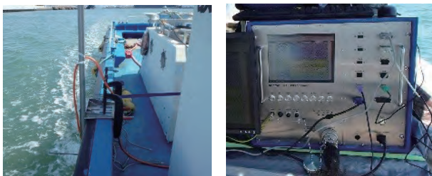
写真1 SES2000の艦装状況(左)とモニター(右)
